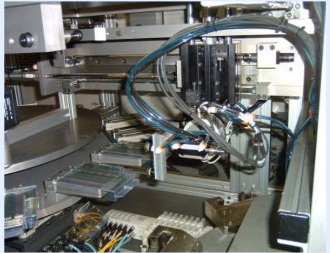
Módulo de transferencia de partes con movimiento X-Y-Z-R
